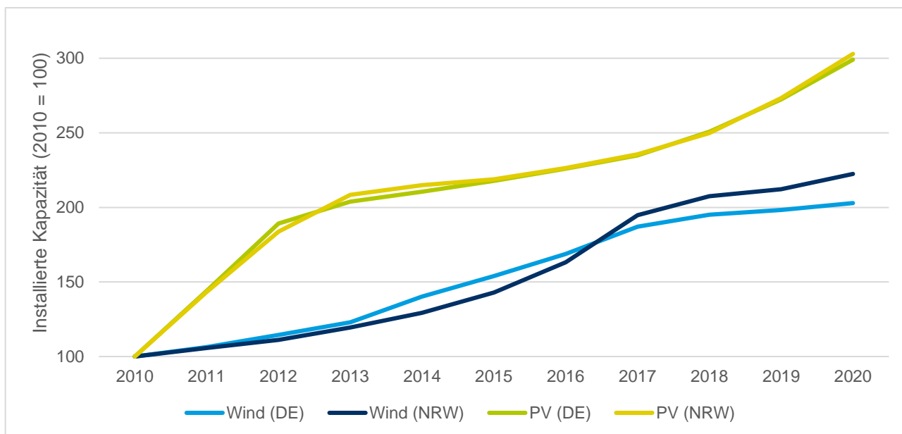
Abbildung 2: Entwicklung der Wind- und PV-Kapazitäten in Deutschland und NRW im Vergleich zu 2010
