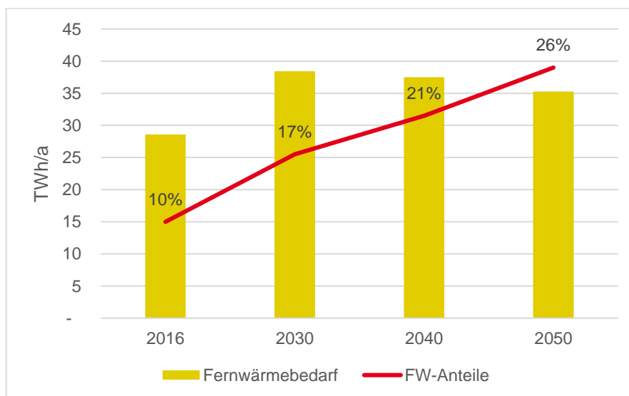
Abbildung 3: Entwicklung des Fernwärmebedarfs in Nordrhein-Westfalen sowie des Fernwärmeanteils am Gesamtwärmebedarf in Nordrhein-Westfalen gemäß KWK-Potenzialstudie 18
