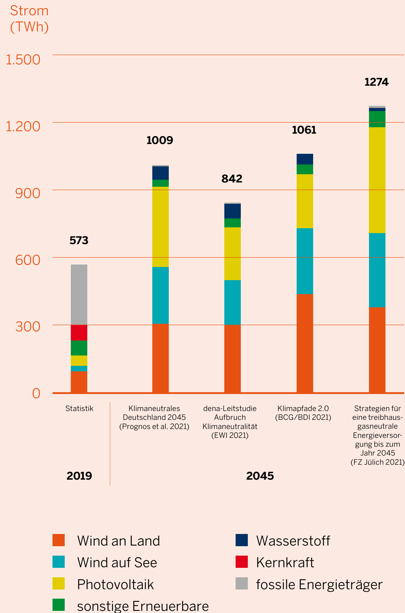
Abbildung 16: Stromerzeugung nach Energieträgern Inländische Stromerzeugung nach Energieträgern in den Jahren 2019 und 2045 Quelle: SC14climate.NRW 2022, Quantitativer Vergleich aktueller Klimaschutzenszenarien für Deutschland, Wuppertal
