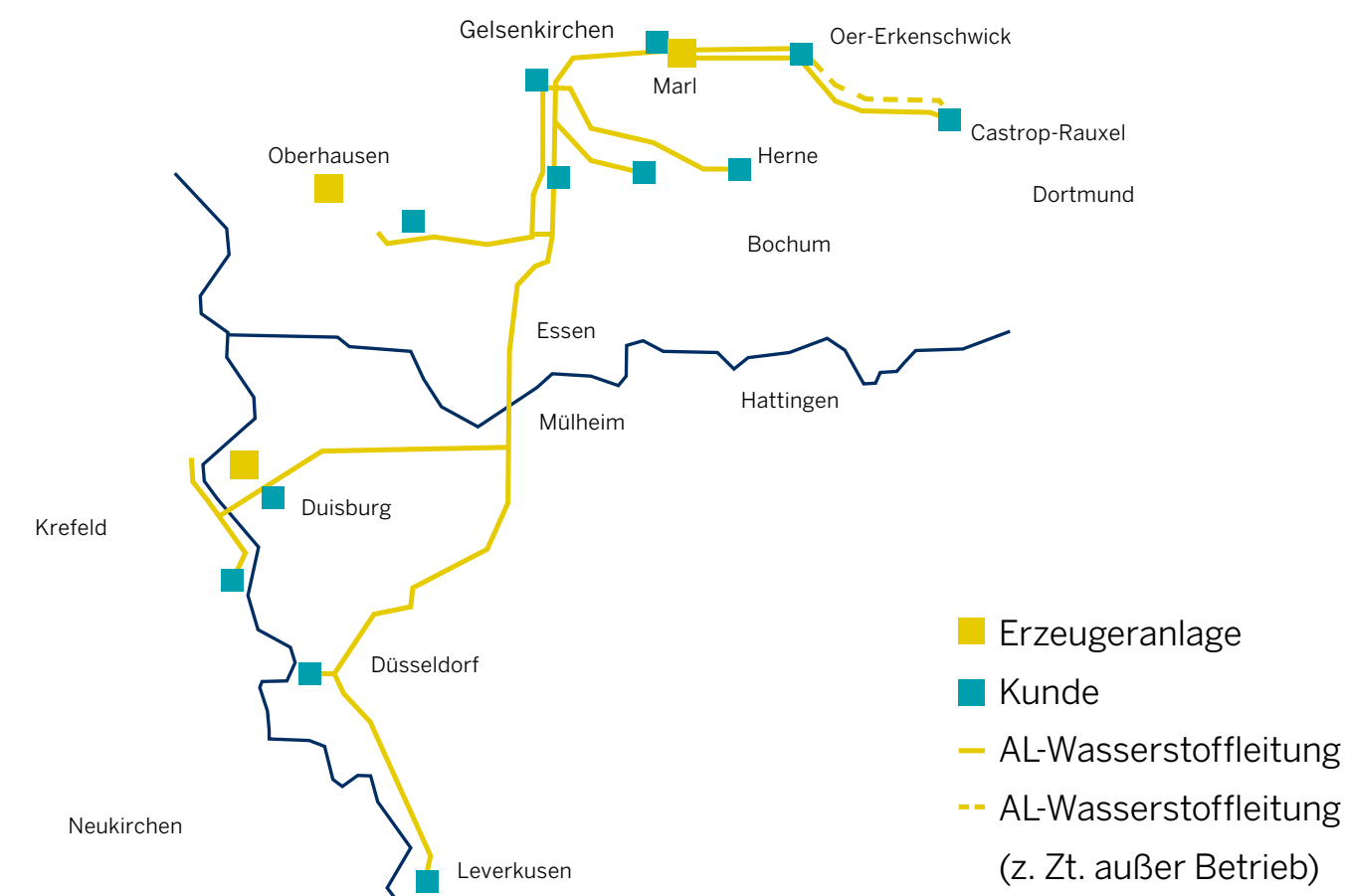
Abbildung 09: Das derzeit größte Wasserstoffnetz in Deutschland befindet sich in Nordrhein-Westfalen, wird von Air Liquide betrieben und ist 240 Kilometer lang.
